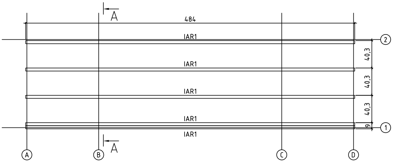
FOUNDATION - FUNDAMENT - FONDATION
