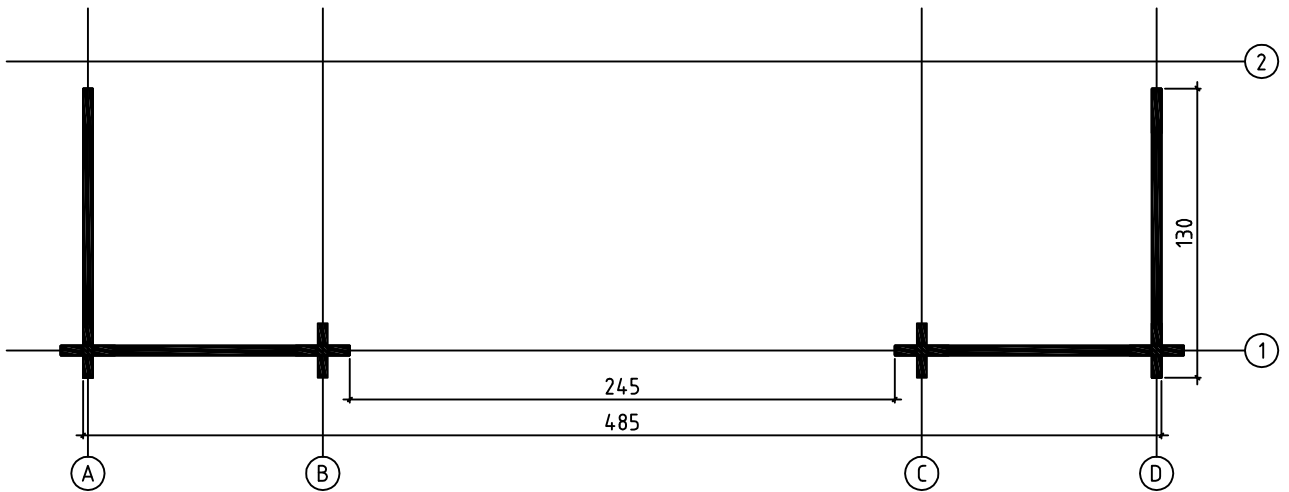
GROUNDPLAN - GRUNDPLAN - PLAN DE MASSE
